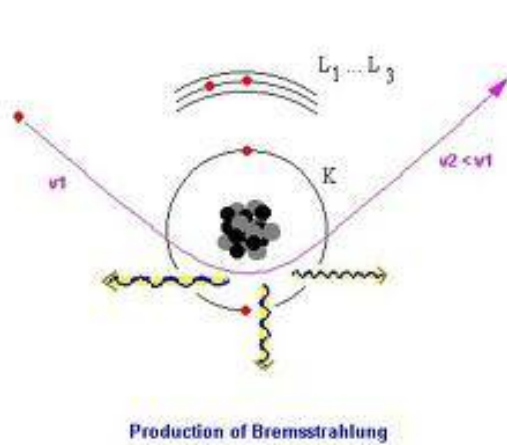
Bremsstrahlung radiation
