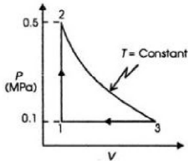
P-V diagram .
