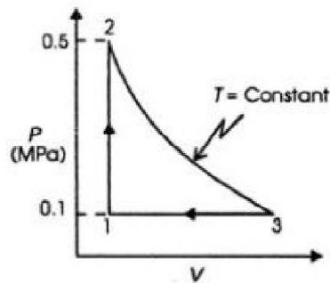
P-V diagram .
